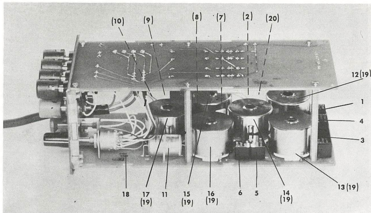
AFB 1.4.4 - GEDRUKTE SCHAKELING
