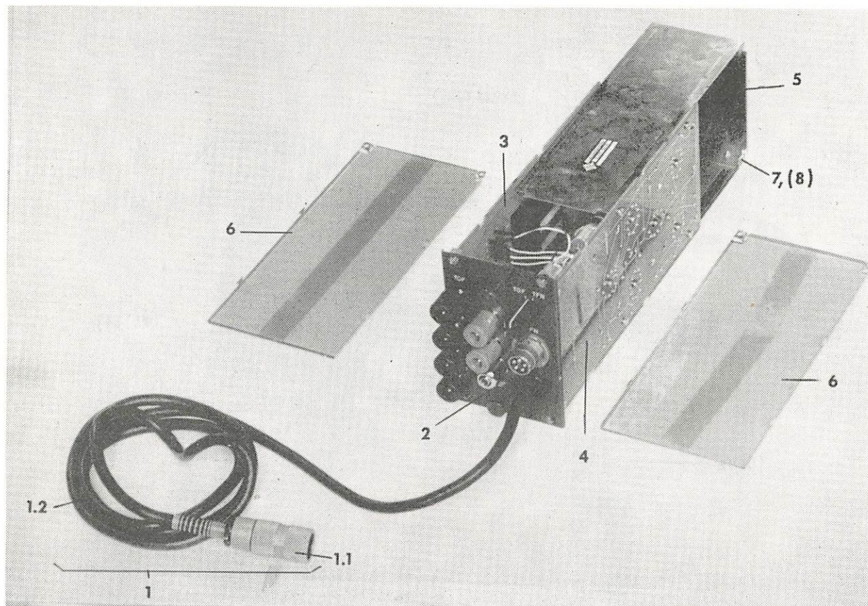
Afb. 1.4 - AANPASSINGSEENHEID
