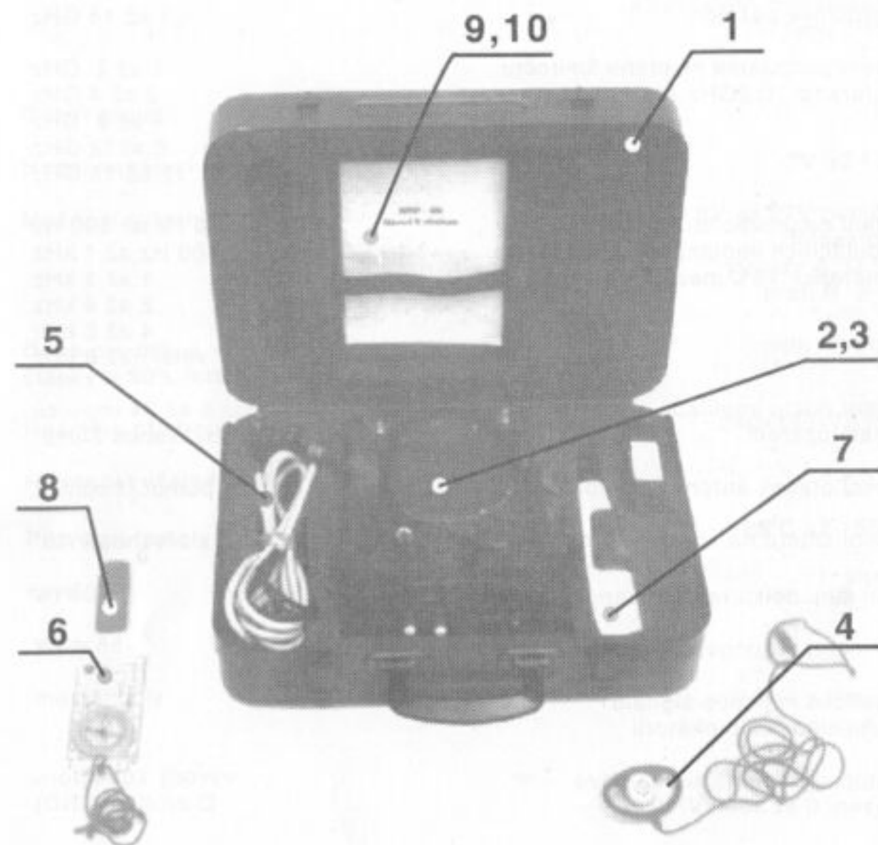
Obr. 1 PÁTRAČ MRP-4M KOMPLETOVANÝ
