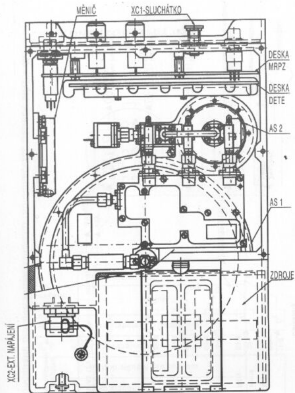
ZÁSTAVBA PÁTRAČE MRP-4M
