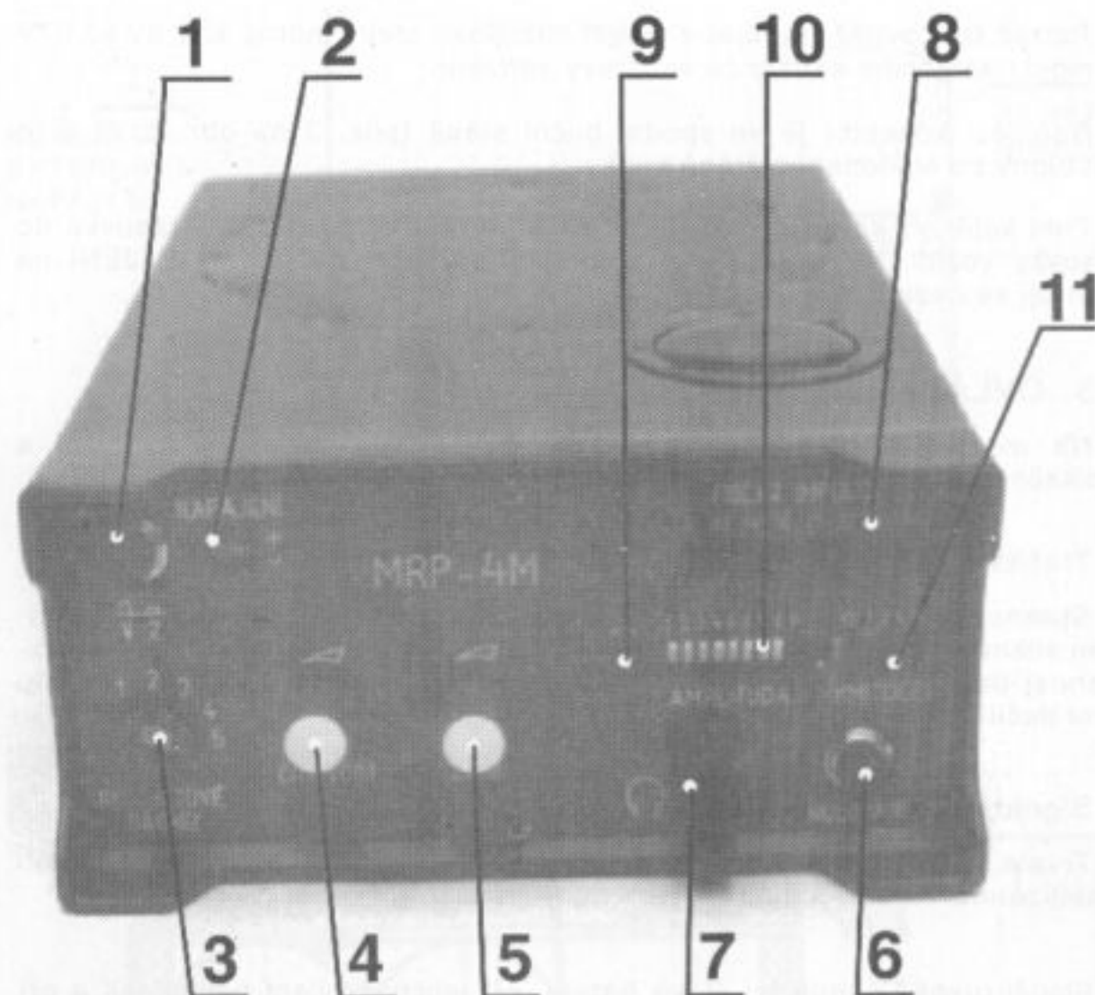
Obr. 3 - OVLÁDACÍ PANEL PÁTRAČE
