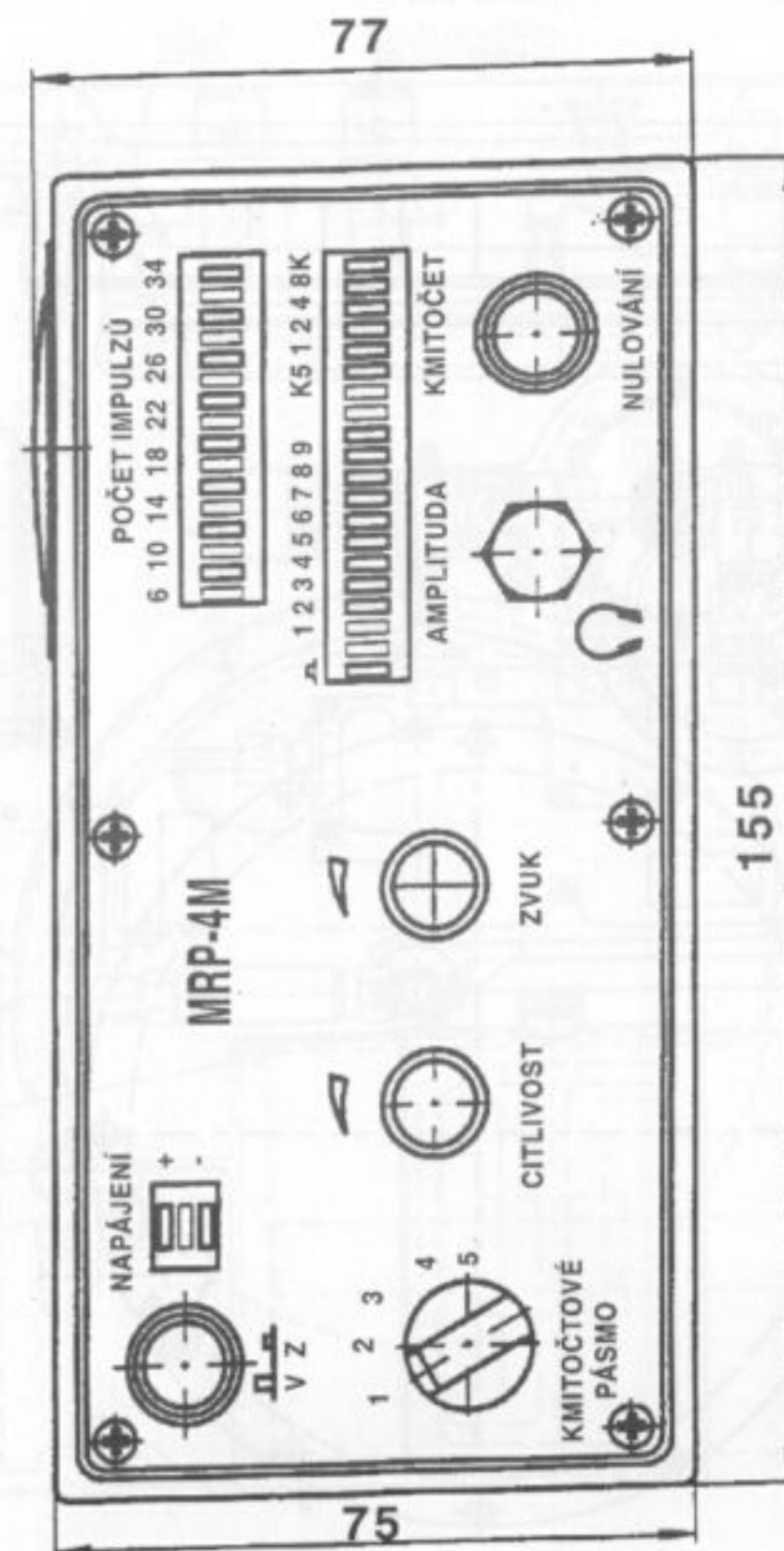
Ovládací panel pátrače
